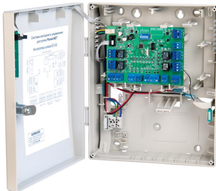
Рисунок 1. Внешний вид модуля сопряжения в открытом корпусе
