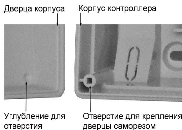
Рисунок 8. Схема «жесткого» крепления дверцы к корпусу модуля сопряжения
