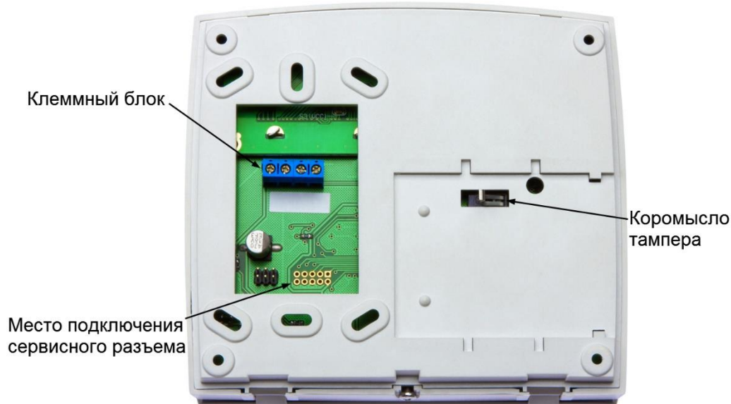
Рисунок 2. Вид клавиатуры АКД-01 сзади
