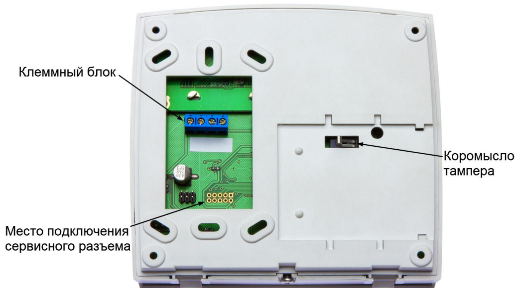
Рисунок 2. Вид клавиатуры АКD-01 сзади
