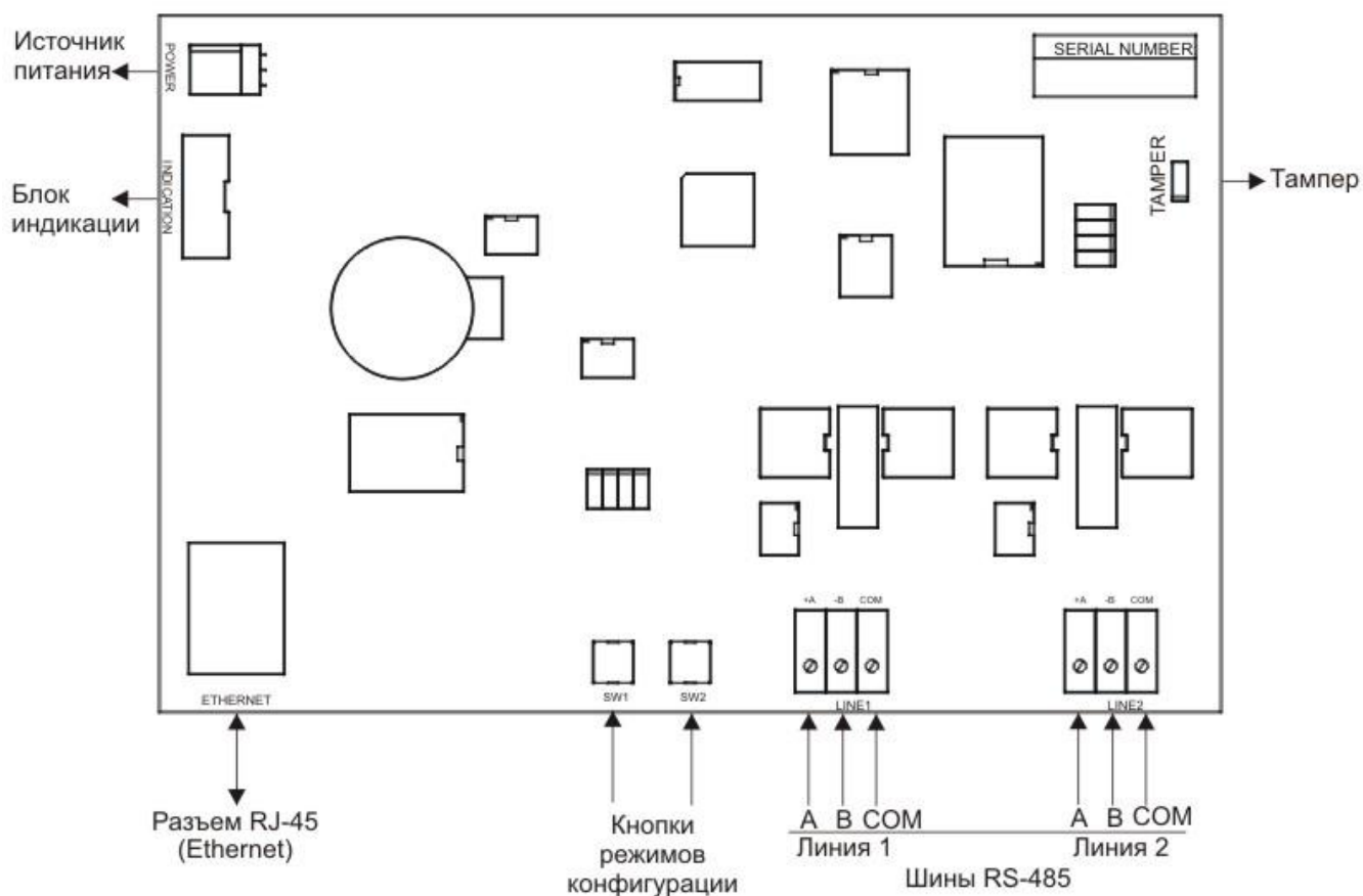
Рисунок 8. Плата шлюза с основными элементами.
