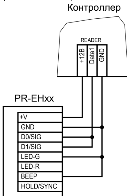
Рисунок 6. Подключение считывателя в режиме Touch
