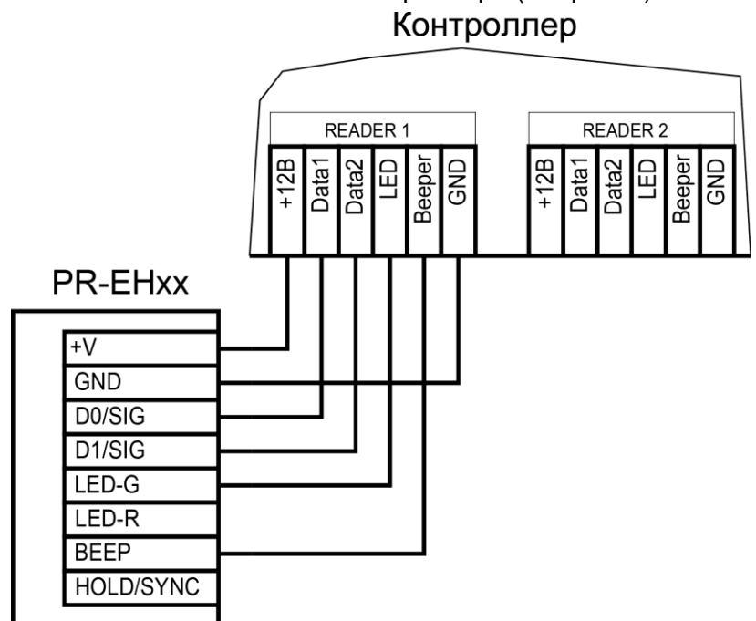
Рисунок 7. Подключение считывателя в режиме Wiegand
