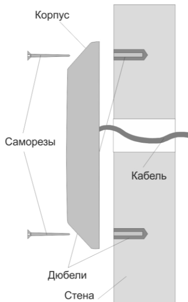
Рисунок 2. Крепление PR-EH03
