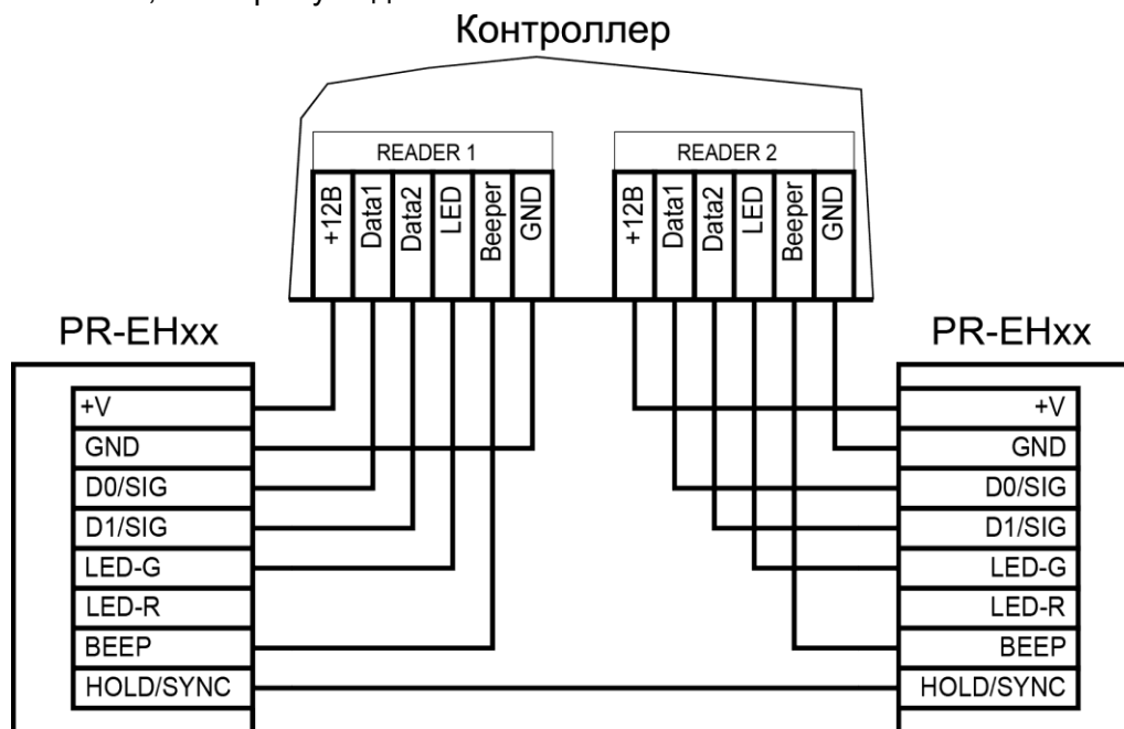
Рисунок 3. Синхронизация считывателей, подключенных в режиме Wiegand
