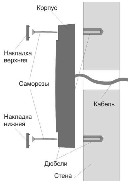
Рисунок 4. Крепление считывателя PNR-P19
