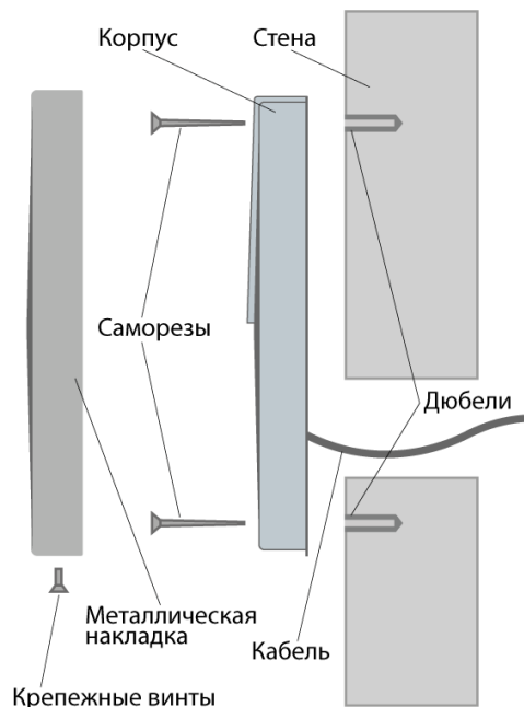
Рисунок 2. Крепление считывателя PNR-P15
