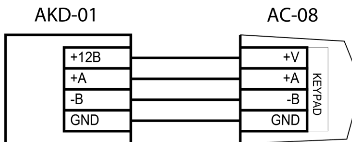
Рисунок 3. Схема подключение клавиатуры к охранному контроллеру
