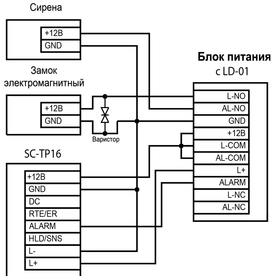
Рисунок 6. Управление замком и сиреной через дешифратор
