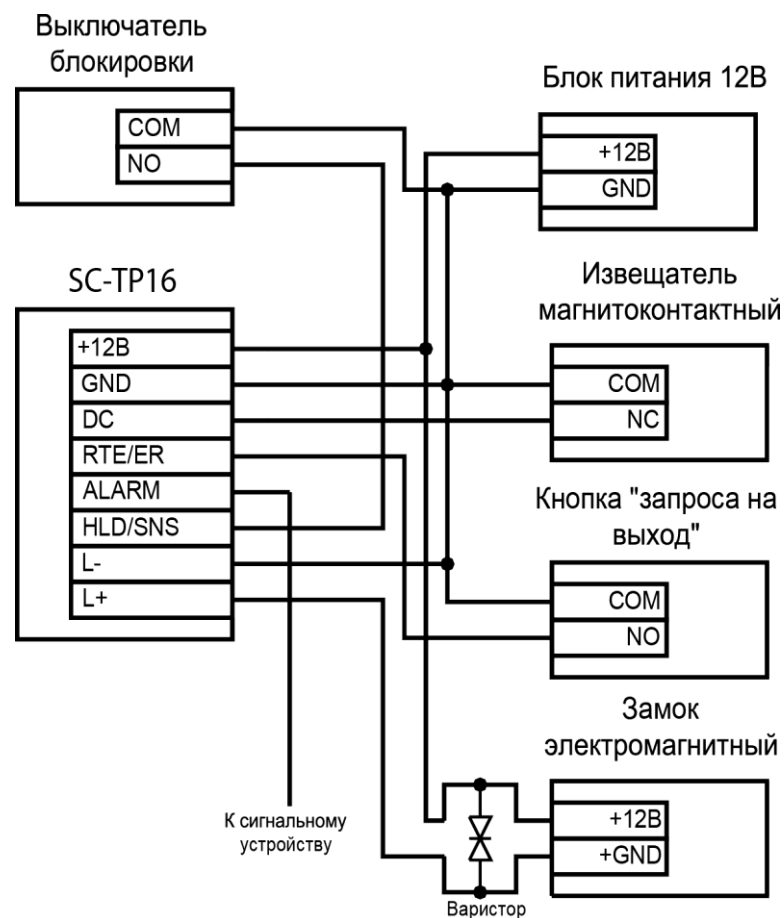
Рисунок 3. Подключение контроллера в заводской конфигурации
