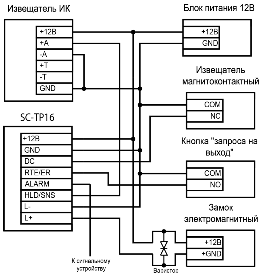
Рисунок 4. Подключение охранного датчика
