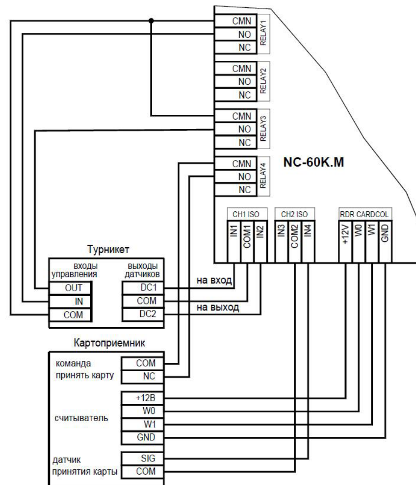
Рисунок 17. Схема подключения турникета и картоприемника
