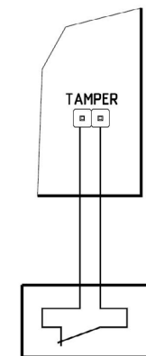
Рисунок 25. Подключение тампера корпуса
