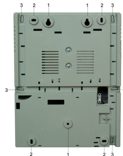
Рисунок 3. Монтажные отверстия
