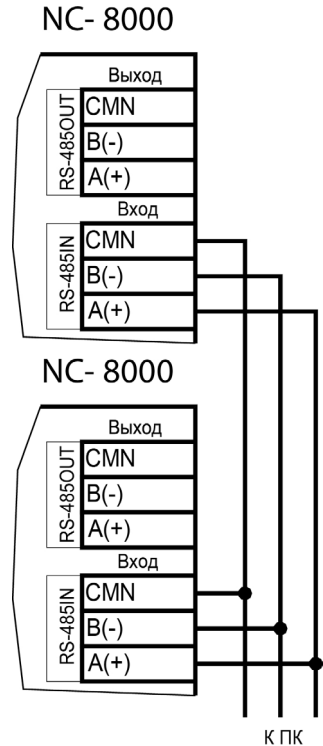
Рисунок 29. Схема соединения контроллеров по топологии «Звезда»
