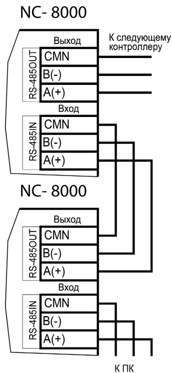
Рисунок 28. Схема соединения контроллеров по топологии «Шина»
