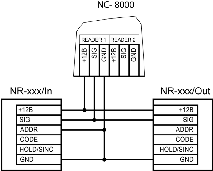
Рисунок 10. Схема подключения считывателей серии NR к контроллеру одним кабелем
