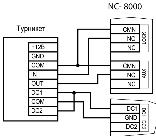
Рисунок 16. Схема подключения контроллера к турникету
