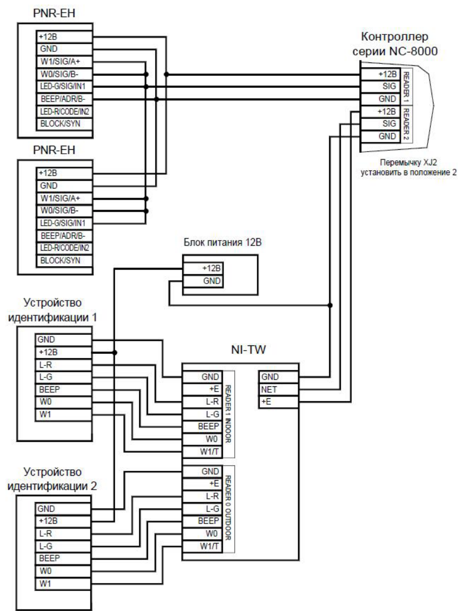
Рисунок 9. Схема подключения 2 считывателей с интерфейсом Parsec и 2 устройств идентификации с интерфейсом Wiegand
