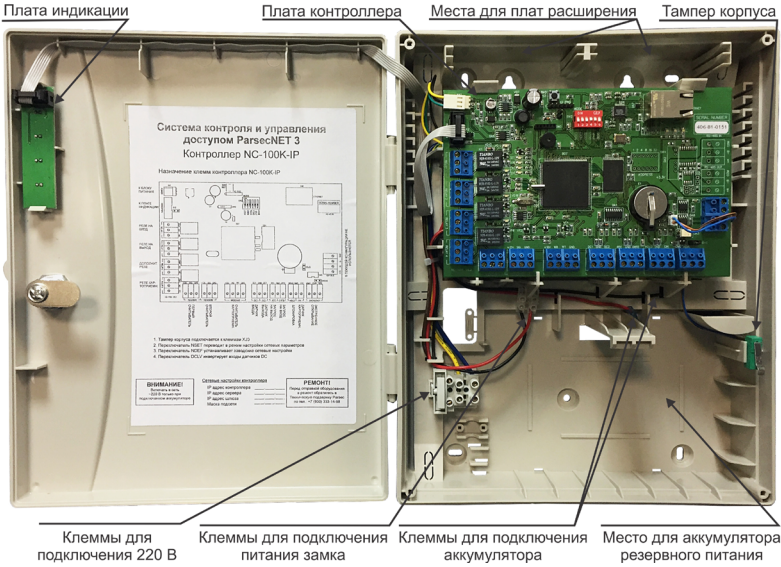
Рисунок 1. Открытый корпус с платой контроллера
