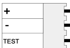
Рисунок 3. Назначение контактов разъема POWER
