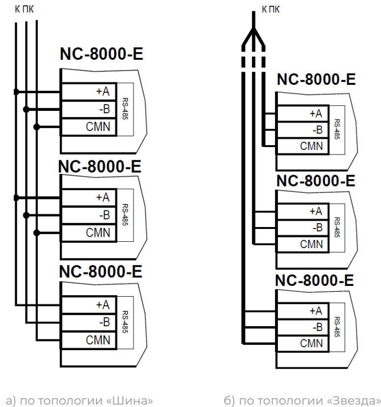
Рисунок 8. Схема соединения контроллеров
