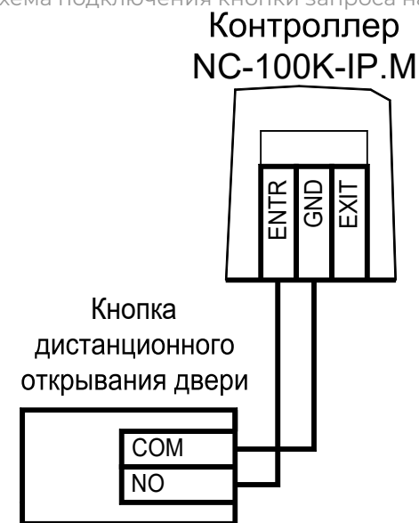
Рисунок 14. Схема подключения кнопки удаленного открывания двери
