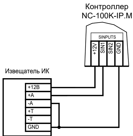
Рисунок 18. Схема подключения охранного датчика с контролем состояния линии
