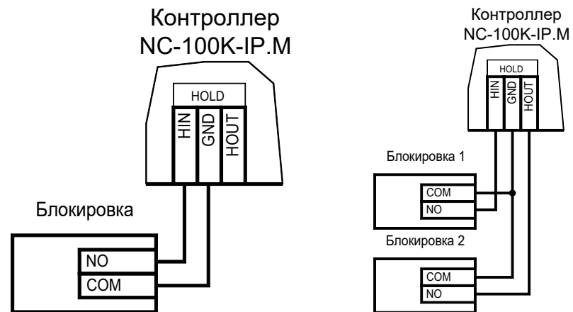
Рисунок 20. Схемы подключения блокировки контроллера
