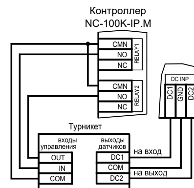
Рисунок 16. Схема подключения 1 датчика проворота турникета
