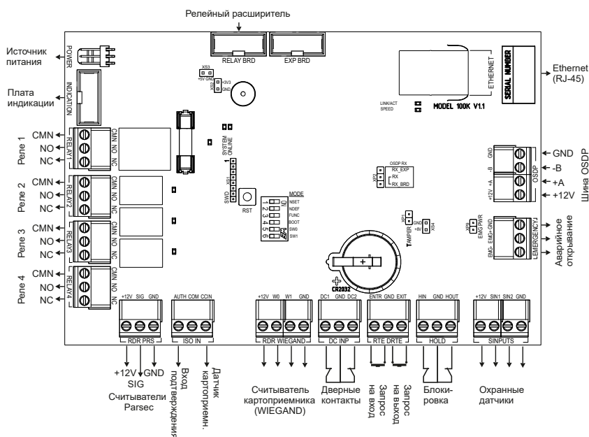
Рисунок 2. Схема платы контроллера NC-100K-IP.M
