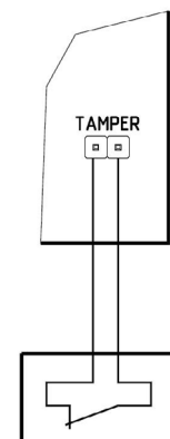
Микровыключатель
