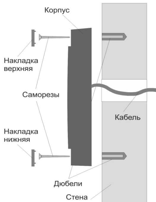
Рисунок 2. Крепление считывателя
